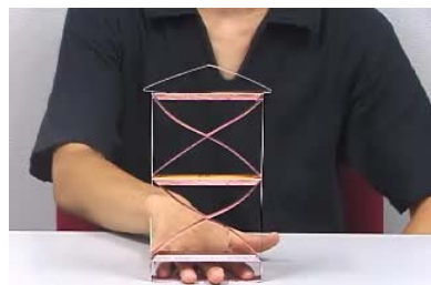
①. 1階と2階に「筋交い」を入れて実験
