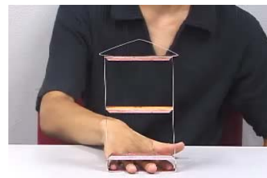
③. 1階と2階の「筋交い」を外してて実験
