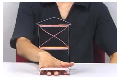
②. 1階の「筋交い」を外して実験
